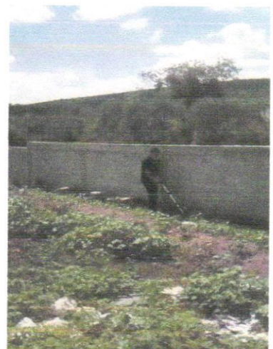
Vista de barda de panteón donde se observa el muro de block, cadena de desplante, cadena de cerramiento, castillos y cimiento de piedra braza
