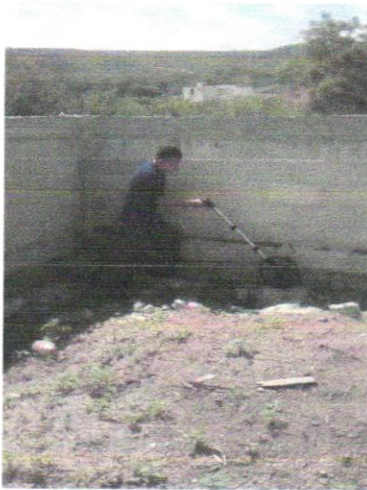
Vista de barda de panteón donde se observa el muro de block, cadena de desplante, cadena de cerramiento, castillos y cimiento de piedra braza
